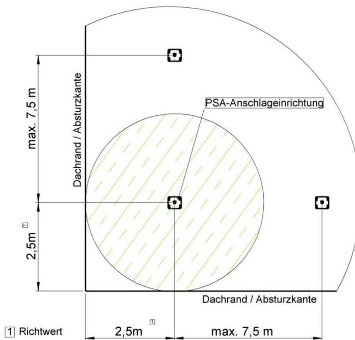
Positionsskizze Dach
